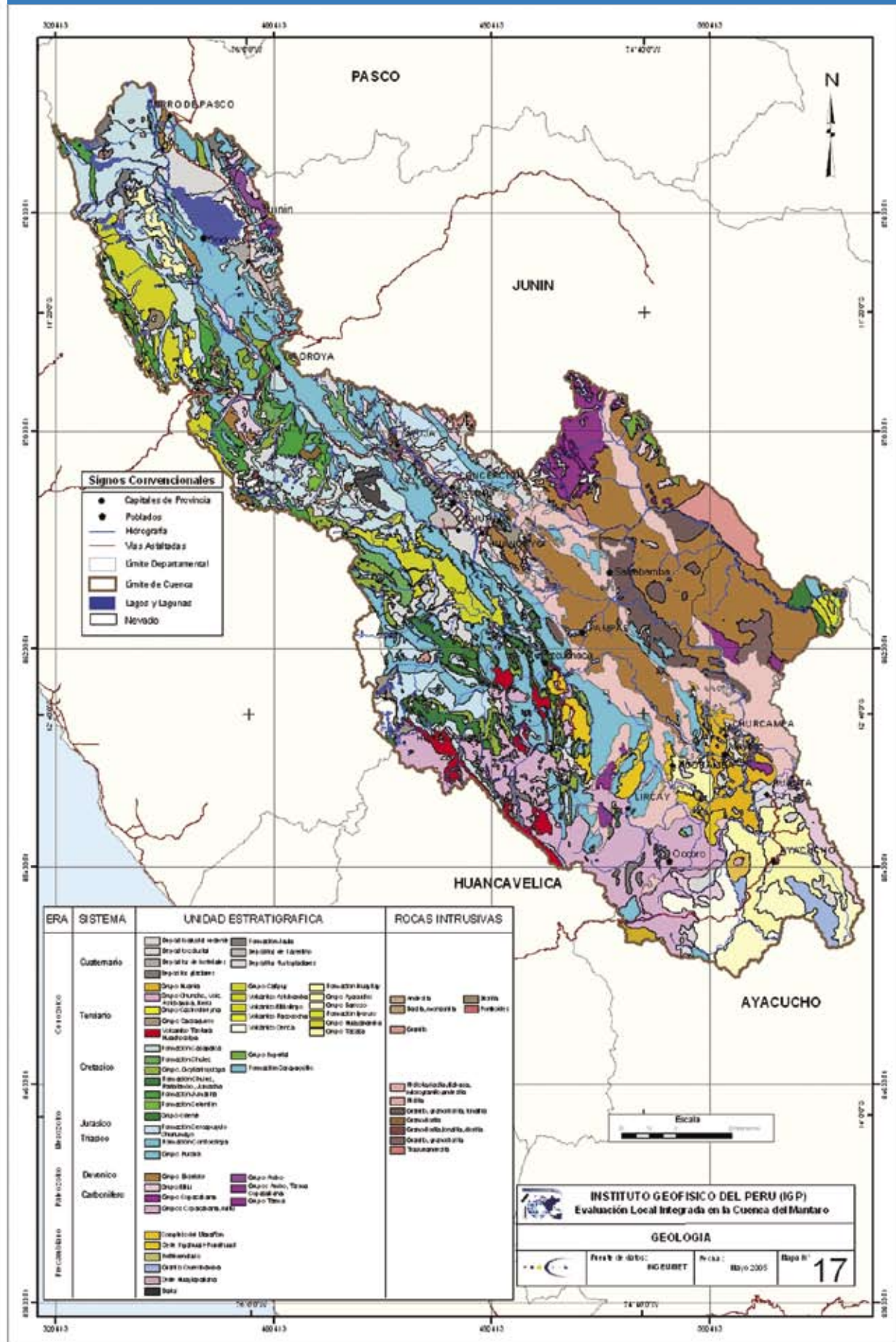
Mapa Nro. 17 Geología
